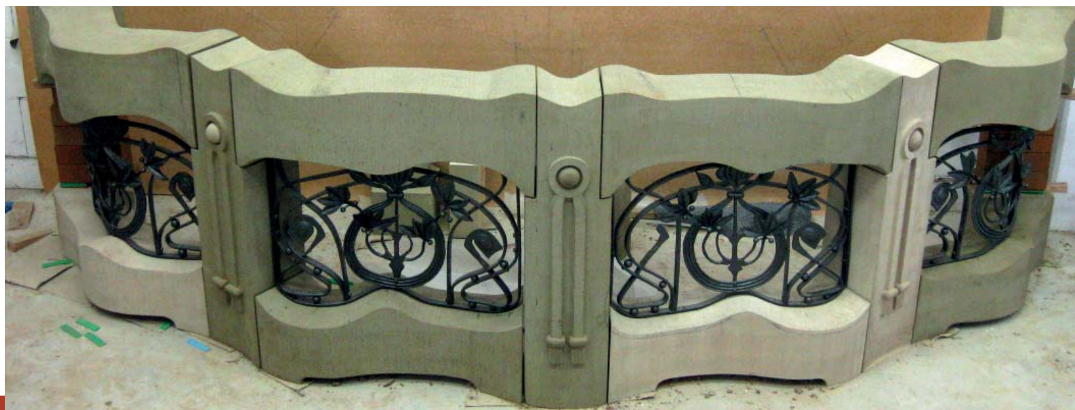
Fertige Brüstung in der Werkstatt mit Aufriss der Draufsicht im Hintergrund.
